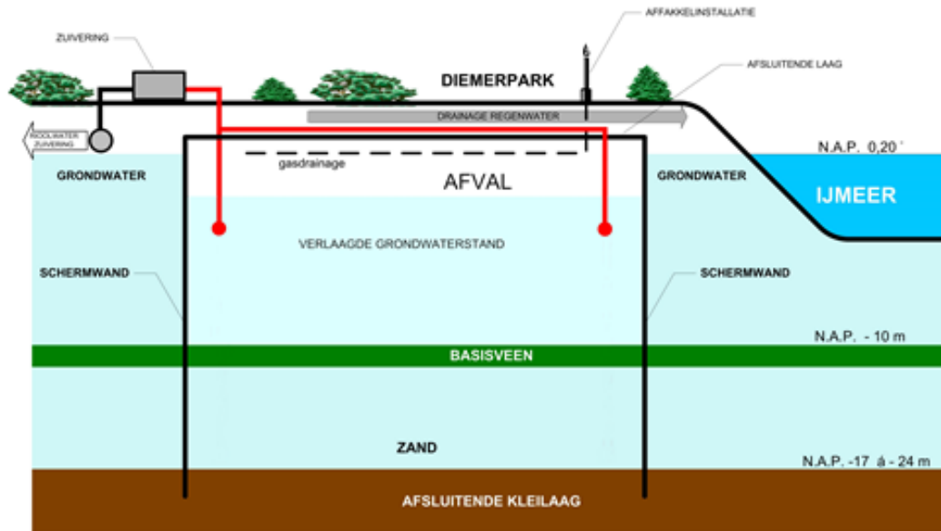
Figuur 1: Doorsnede Saneringsaanpak
